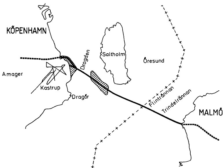
Figur 1. Öresundsförbindelsens sträckning.
